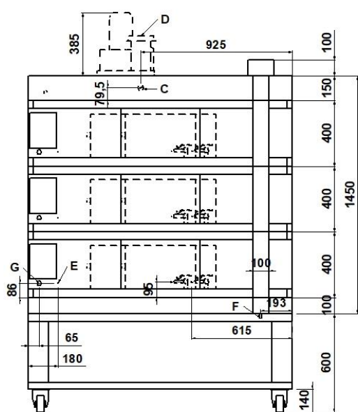
VISTA POSTERIORE
