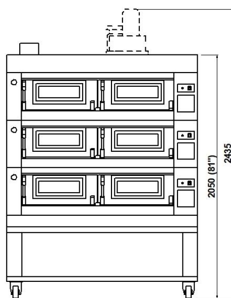
VISTA FRONTALE
