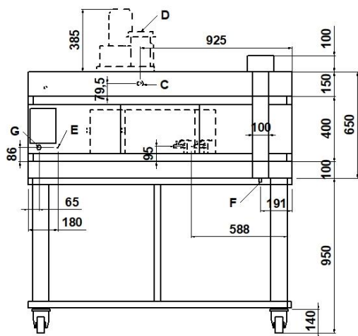
VISTA POSTERIORE
